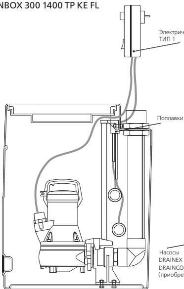
Комплект обвязки для установки DRAINBOX 300 1400 TP KE FL
