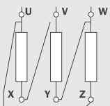
Соединение Звезда
