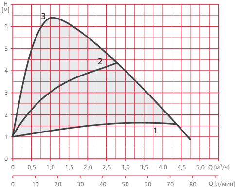
Пропорциональное давление
