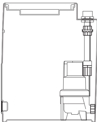
Комплект обвязки для установки DRAINBOX 300 1400 TP KE FL
