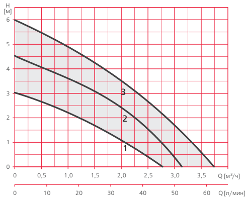
Постоянная скорость
