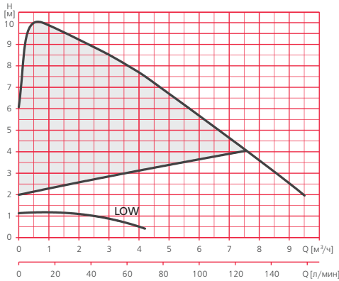
Пропорциональное давление
