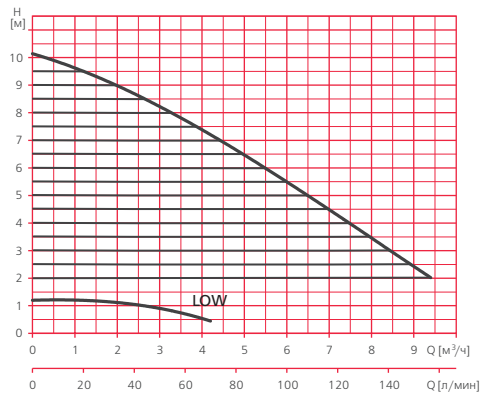
Постоянное давление
