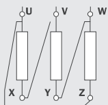
Соединение Треугольник
